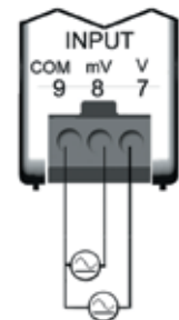
Voltage Input
